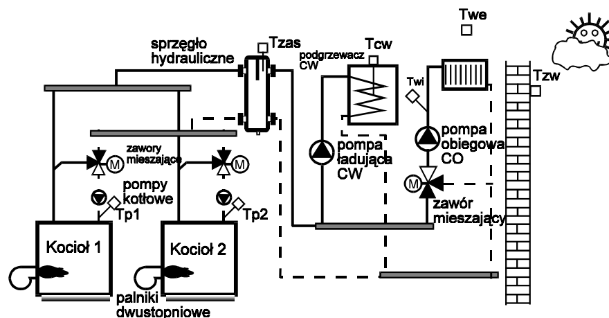
Rys. 1a Układ U1 sterowany regulatorem w wersji KMCS
