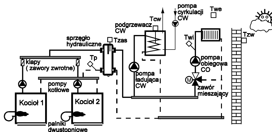
Rys. 1b Układ U2 sterowany regulatorem w wersji KMCS
