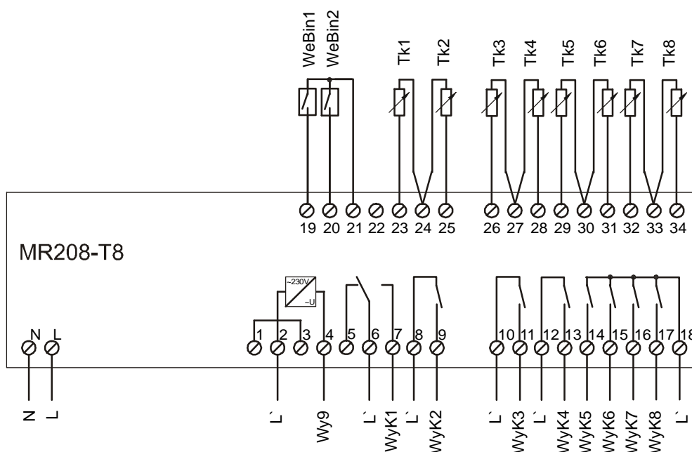
Schemat połączeń elektrycznych MR208-T8.
