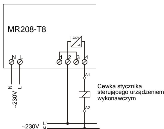
Schemat podłączenia cewki przekaźnika/stycznika:
