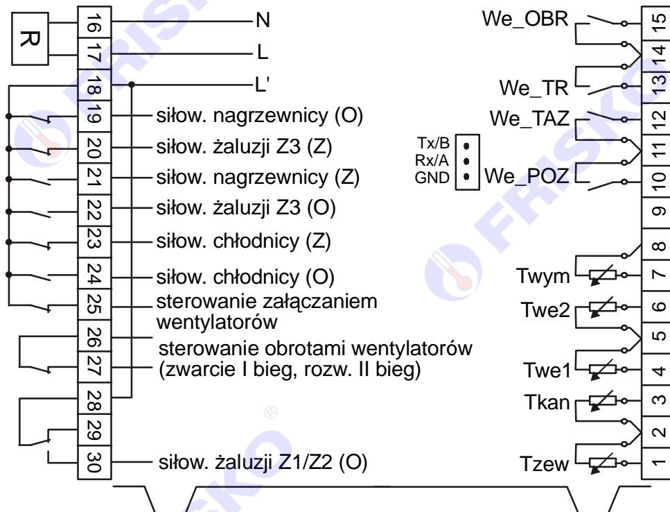
Schemat połączeń elektrycznych RX910-KLIMAX (montaż tablicowy - widok złącz na tylnej ścianie regulatora)
