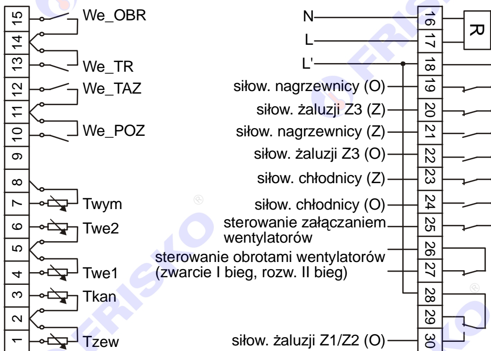
Schemat połączeń elektrycznych RX910-KLIMAX (montaż w cokole - widok złącz cokołu montażowego)
